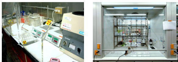
圖二十四 將玻璃櫃門拉下，或增加強化壓克力防護罩，可降低風險
