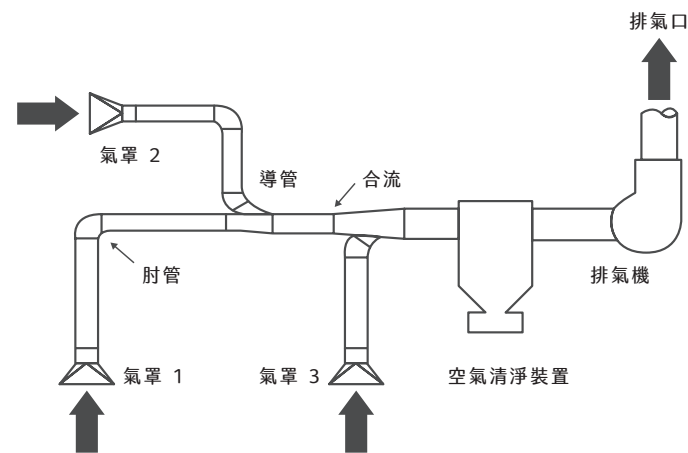
圖四十二 局部排氣裝置概要
