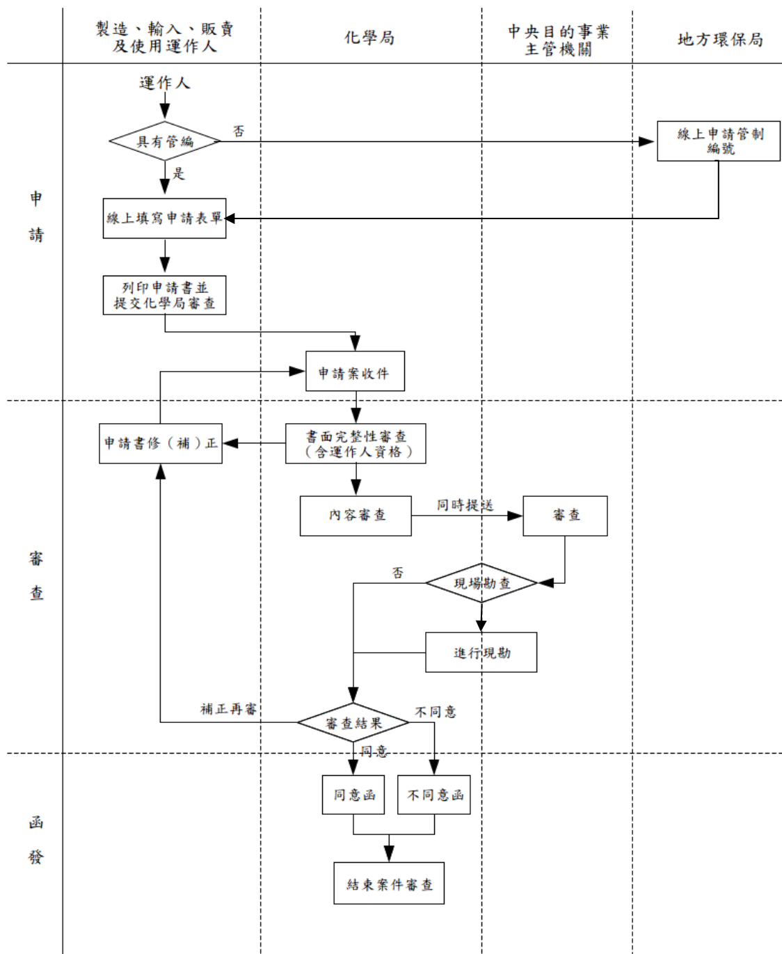
圖、一氧化二氮免添加二氧化硫申請流程圖
