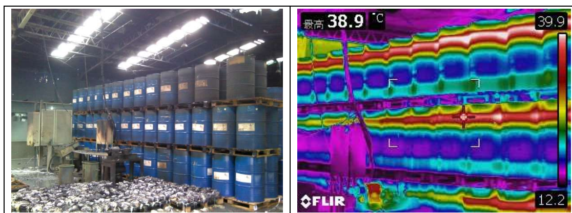
圖 4.2.2 事故現場儲存容器熱影像儀監測作業情形
